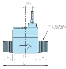
FM0101-S-S-P 表示器なし
