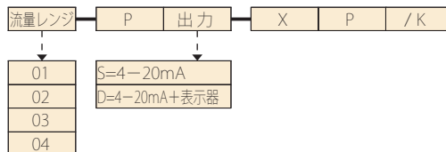
FM31シリーズ (PFA)
