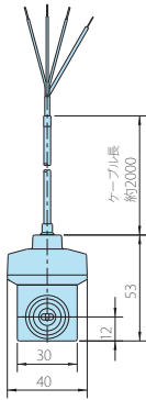
FM0105-S-S-P 表示器なし
